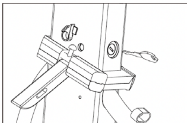
1. Ouvrir le connecteur de pliage,
