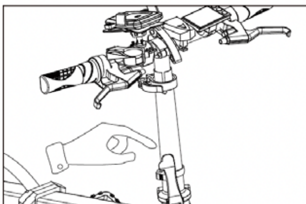
③ Ouvrir le verrou de sécurité
